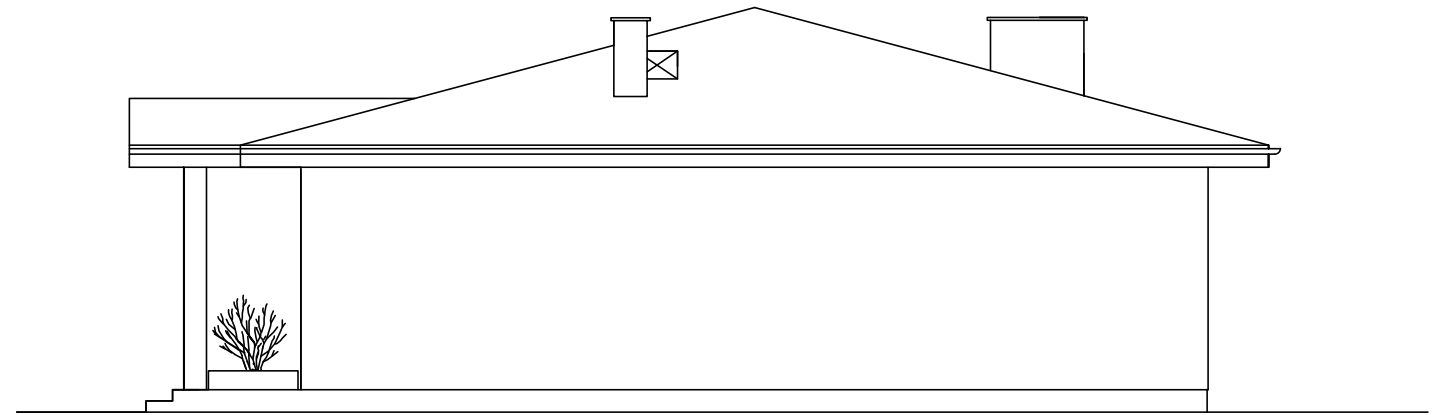
ELEWACJA BOCZNA - PÓŁNOCNA
